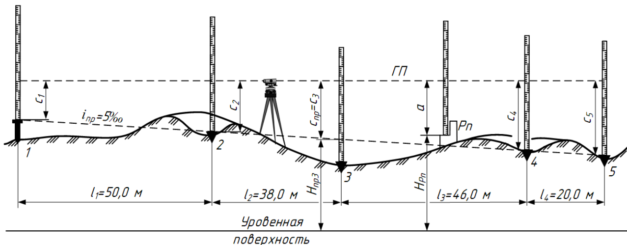
Рисунок 1 Построение линии заданного уклона горизонтальным лучом нивелира
