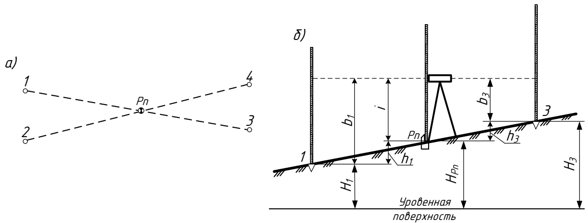
Рисунок 1 Схема нивелирования способом «вперед»
